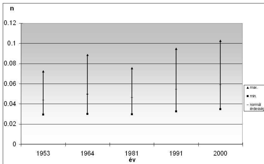
3.24. ábra: A hullámtér hidraulikus érdelesség értékeinek változása a Csordajárás területén
